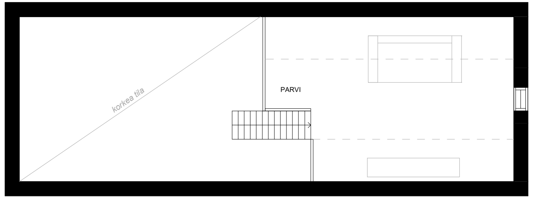
ohjeellinen pohjapiirros parvi
